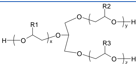
Figura 4: Reprezentarea structurii generale a produsului de reacție dintre glicerol, oxidul de etilenă și oxidul de propilenă (x, y și z sunt numere întregi, R1, R2 și R3 sunt atomi de hidrogen sau grupuri de metil)
