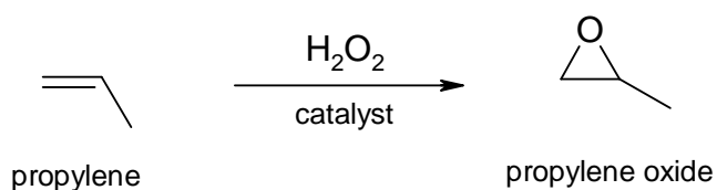
Figura 2: Reacția de epoxidare a propilenei
